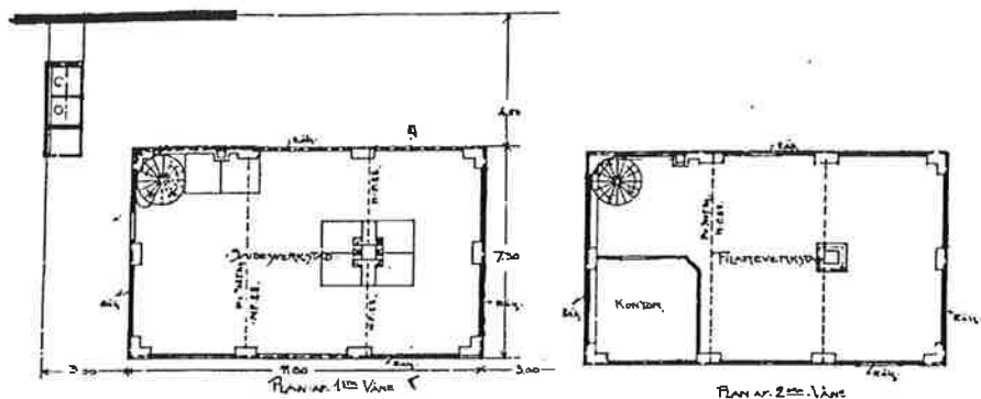
Ritning första och andra våningen från 1902. (GLA)
