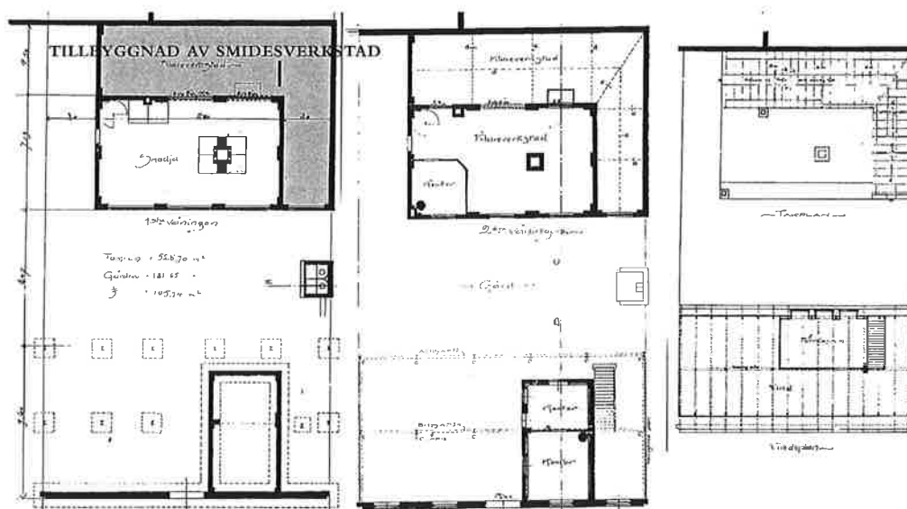
Ritning över "provisionel nybyggnad" med första våning, andra våning samt takplan från 1904.(GLA)
